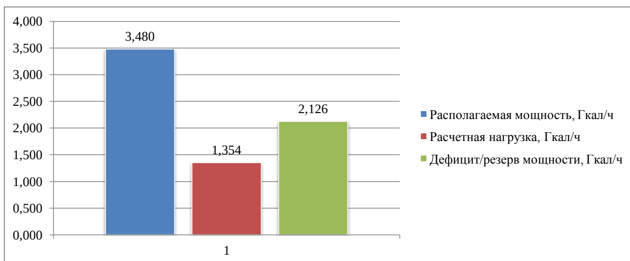
Рис. 2.1 - Балансы тепловой мощности и присоединённой тепловой нагрузки котельной
